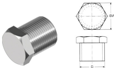
Τάπες αρσενικές WS9630
