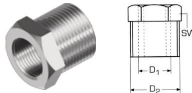
Νίπελ WS9640
