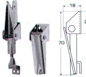
Καταβάτες M8053I
