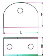
Βάσεις σωλήνα σκάλας M8134
