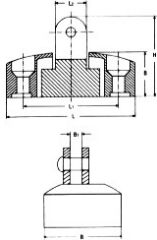
Βάσεις σπαστές για ποτήρι M8573
