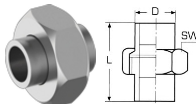
Ρακόρ WS9611S
