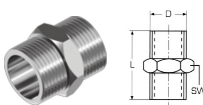
Νίπελ WS9640
