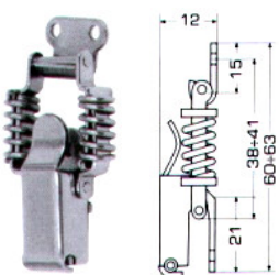
Καταβάτες M8053N
