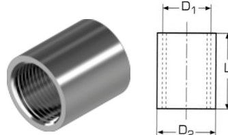
Ρακόρ WS9611S
