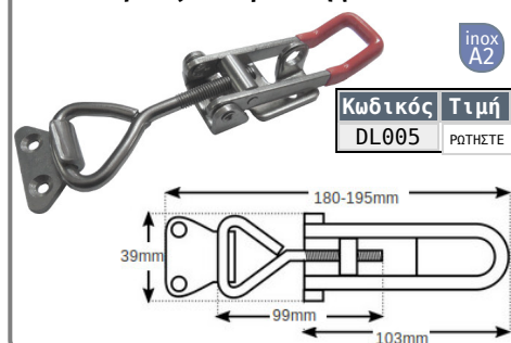
Καταβάτες 8mm με θέση για λουκέτο
