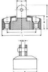
Βάσεις σπαστές για ποτήρι M8573
