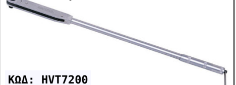
Δυναμόκλειδο 3/4" 200-810Nm
