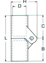
Βάσεις σωλήνα σκάλας M8134
