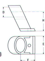
Βάση λοξή 60° διαπερή M8276
