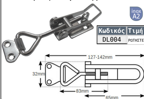
Καταβάτες 6mm με θέση για λουκέτο
