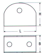
Βάσεις σωλήνα σκάλας M8134
