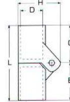
Βάσεις σωλήνα σκάλας M8134
