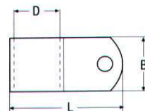
Ταυ σωλήνων πλακέ M8138
